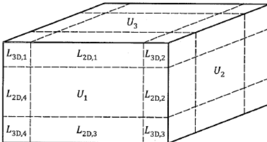
Hình 14 – Vỏ bao che tòa nhà được chia nhỏ theo các mô hình hình học 3-D, 2-D và 1-D
