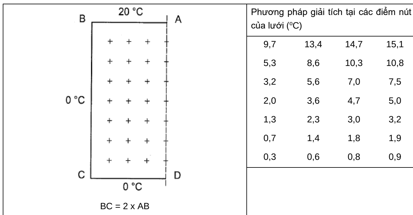
Hình C.1 – Trường hợp kiểm thử tham chiếu 1: So sánh với phương pháp giải tích
