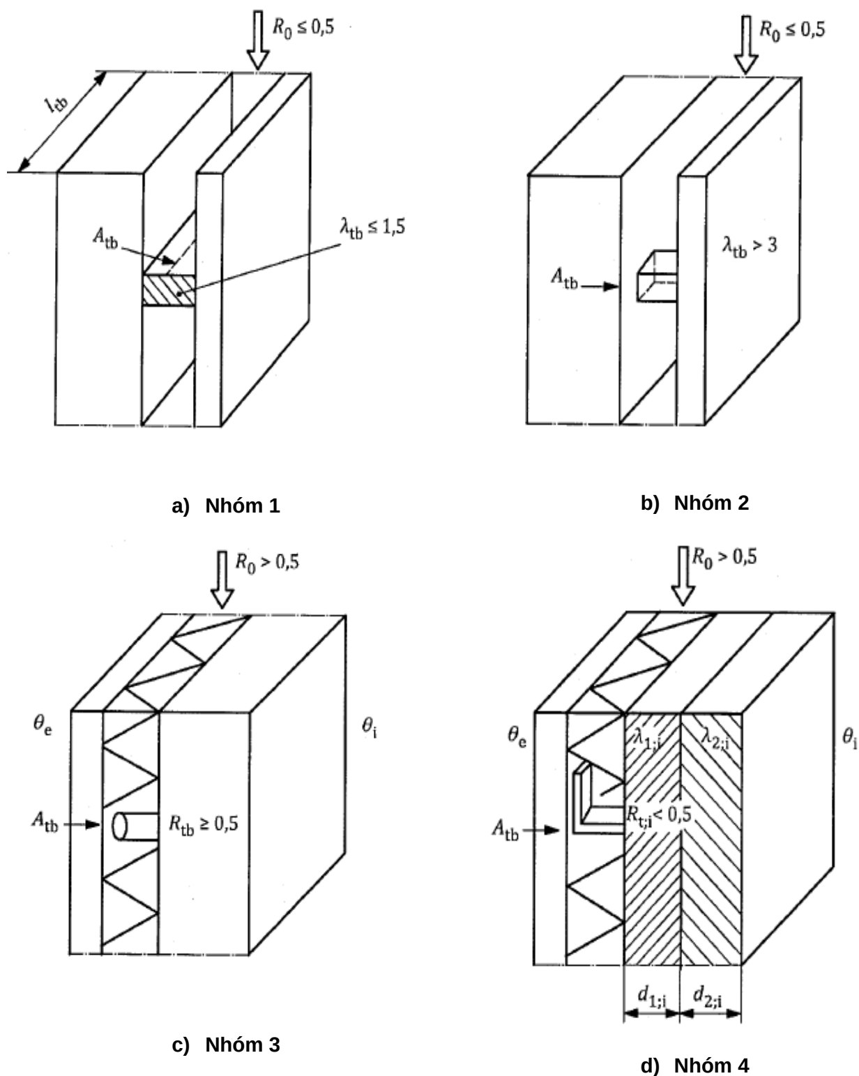
Hình 13 – Các điều kiện cụ thể để hợp nhất các cầu nhiệt tuyến tính và điểm vào trong một lớp gần đồng nhất cho các nhóm nêu trong Bảng 6
