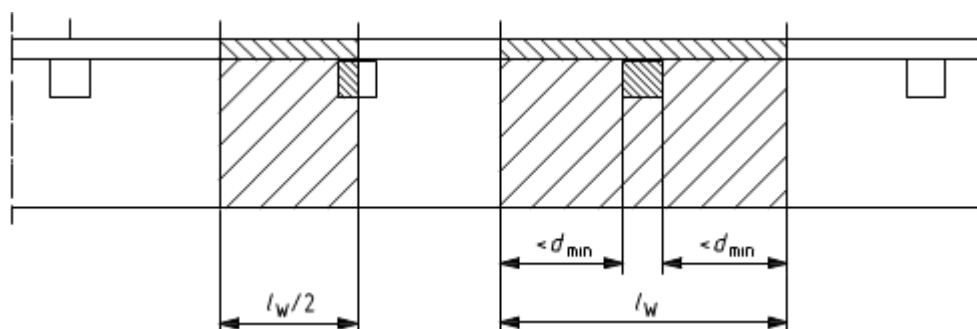
Hình 7 – Vị trí của các mặt cắt phân chia ít nhất bằng d_{min} tính từ phần tử trung tâm trong một mô hình hình học 2-D
